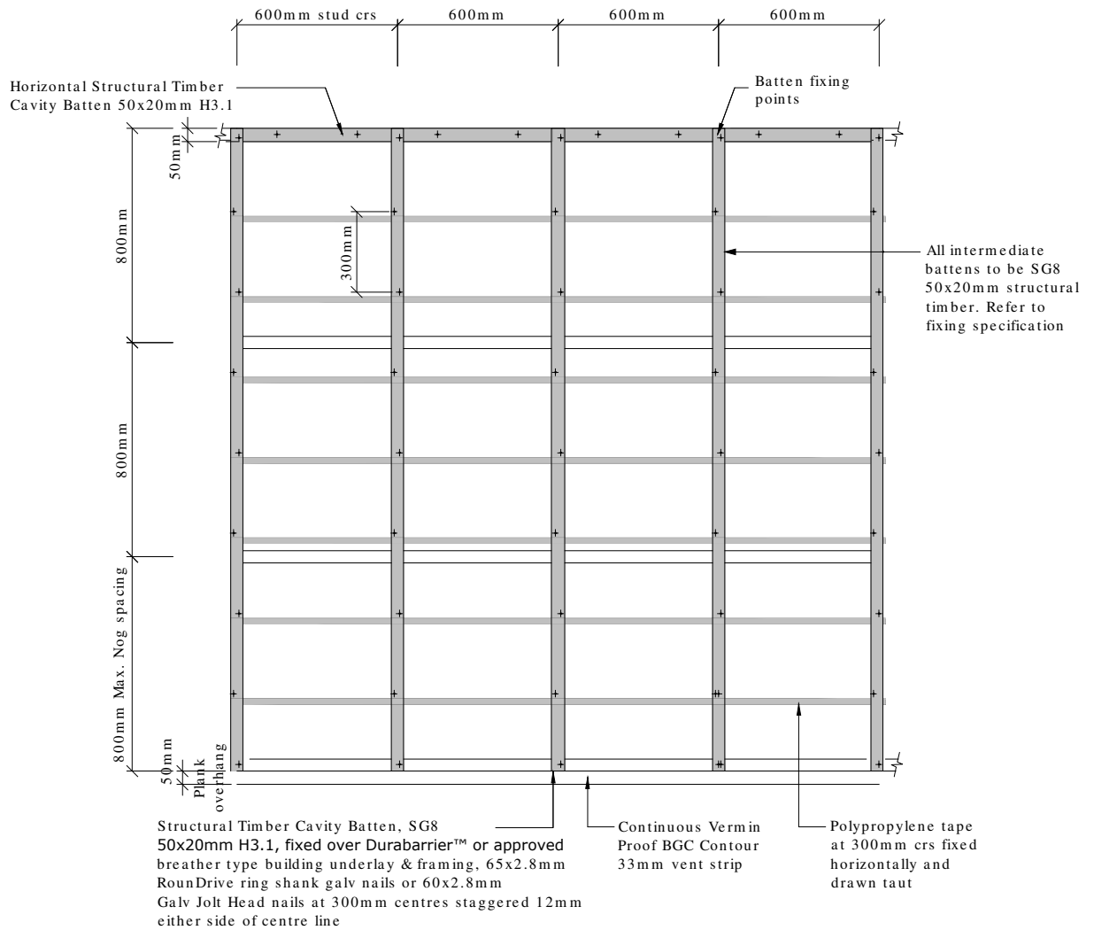
BGC Stratum™ Contour Batten Fixing setout
